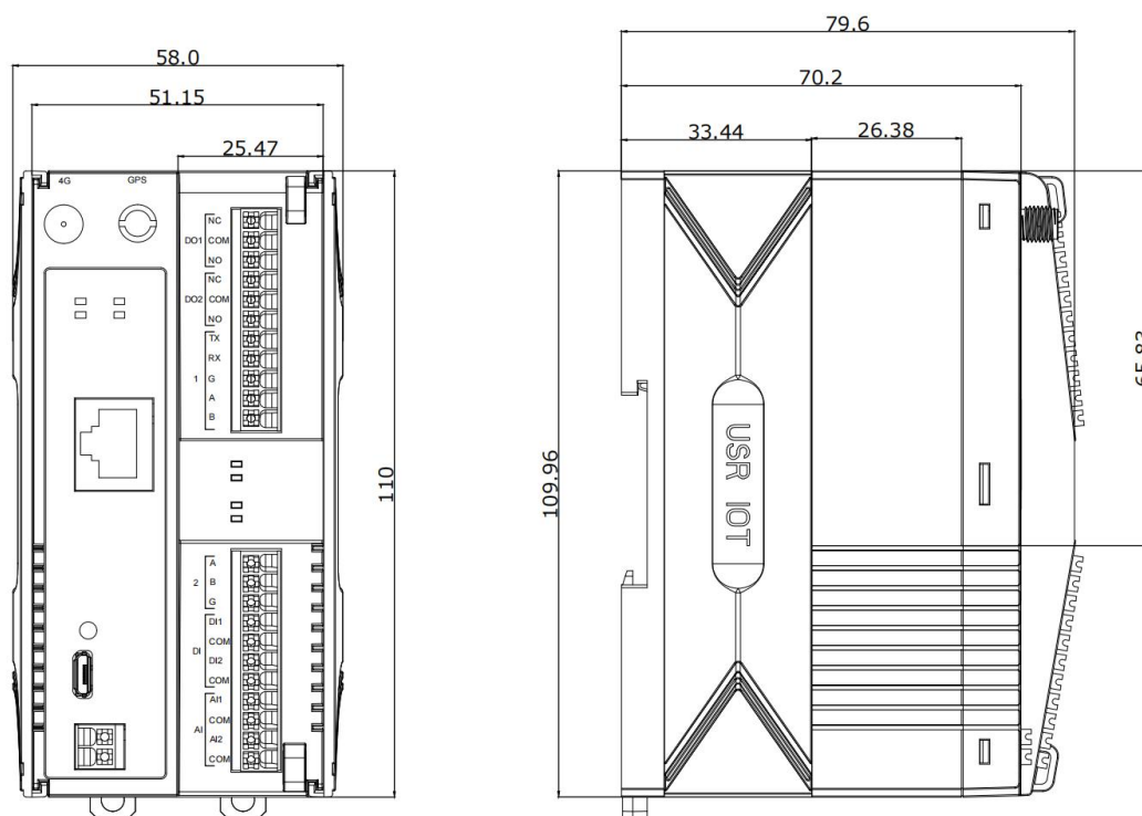
图 1. 尺寸结构图
